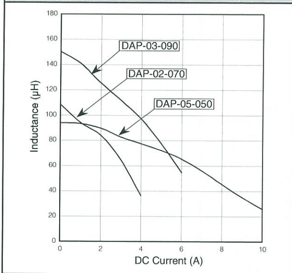
直流重畳特性 (代表例)
